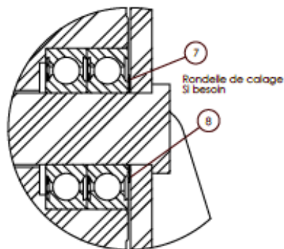
DÉTAIL C Echelle 2:2.5
