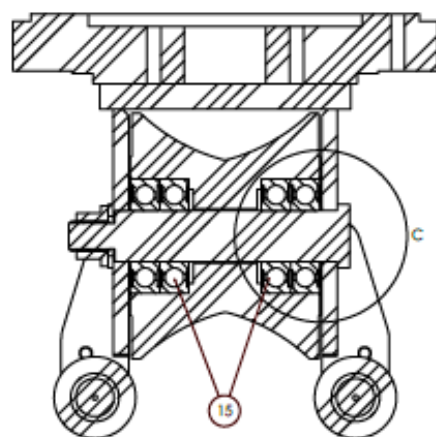
COUPE A-A Echelle 1:2.5
